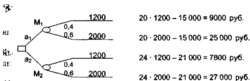
Рис. 4.1. Дерево решений
