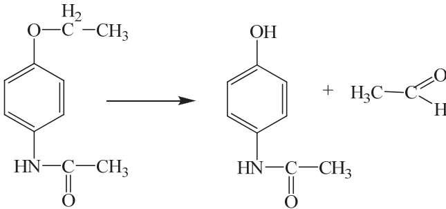
Ֆենացետին
