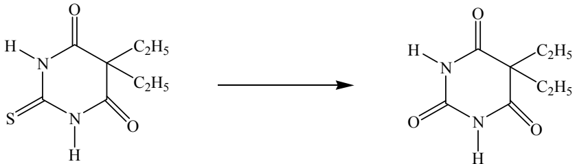
Թիոբարբիտալ
