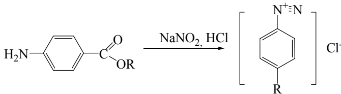
Դիազոնիումային աղ
