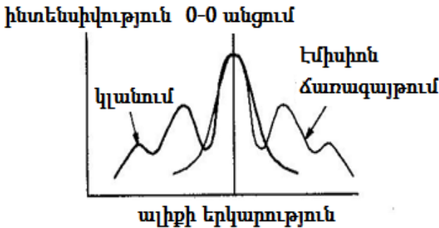
Նկար 36. Կլանման և ֆյուտրեսցենտային ճառագայթման հայելային սպեկտրները:
