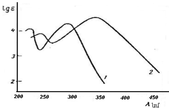
Նկար 23. Զուգորդված արոմատիկ միացությունների կլանման սպեկտրները՝ 1) բենզալացետոնը C_6H_5CH=CHCOCH_3 սպիրտում, 2) 1-ֆենիլպենտադիենալանիլինը C_6H_5CH=CH-CH=CH-CH=N-C_6H_5 սպիրտում:
