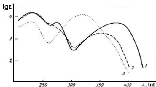
Նկար 26. Նիտրոանիլինների կլանման սպեկտրները հեպտանում՝ 1)օրթո-, 2)մետա-, 3)պարանիտրոանիլին:
