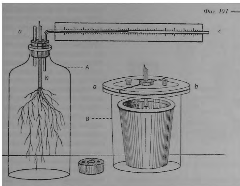
Аппарат с капиллярной трубкой для измерения испарения по всасыванию воды
