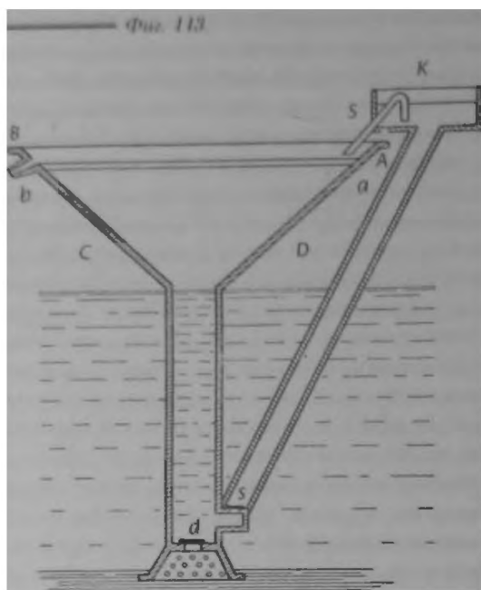
Схема солнечного насоса Мушо
