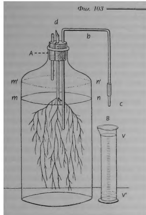
Прибор с сифоном для измерения испарения
